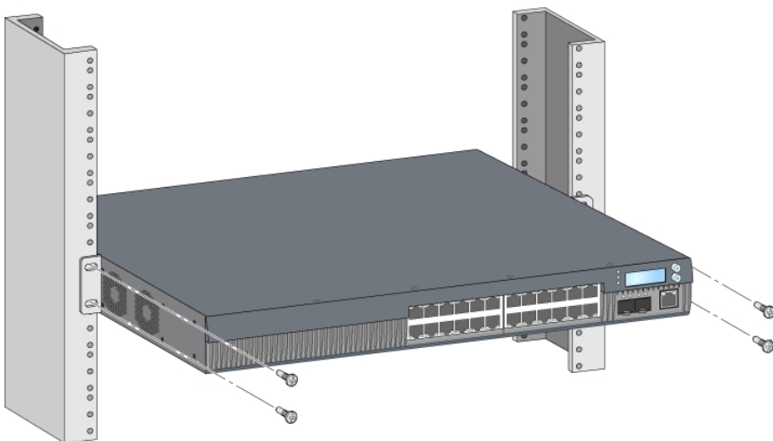
图 10: 中部机架安装
