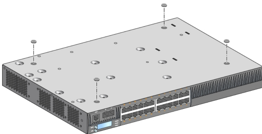
图 11: 连接橡胶脚垫
