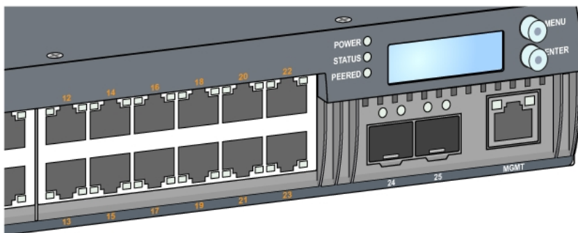
图 4: 10GBase-X 端口、LCD 面板和 LED
