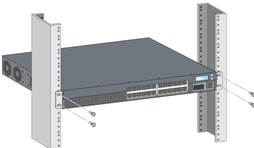
图 8: 前机架安装
