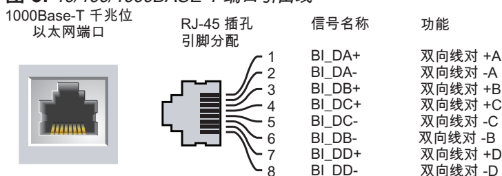
图 3: 10/100/1000BASE-T 端口引出线
