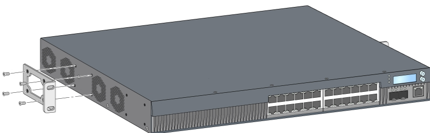
图 9: 中部安装托架
