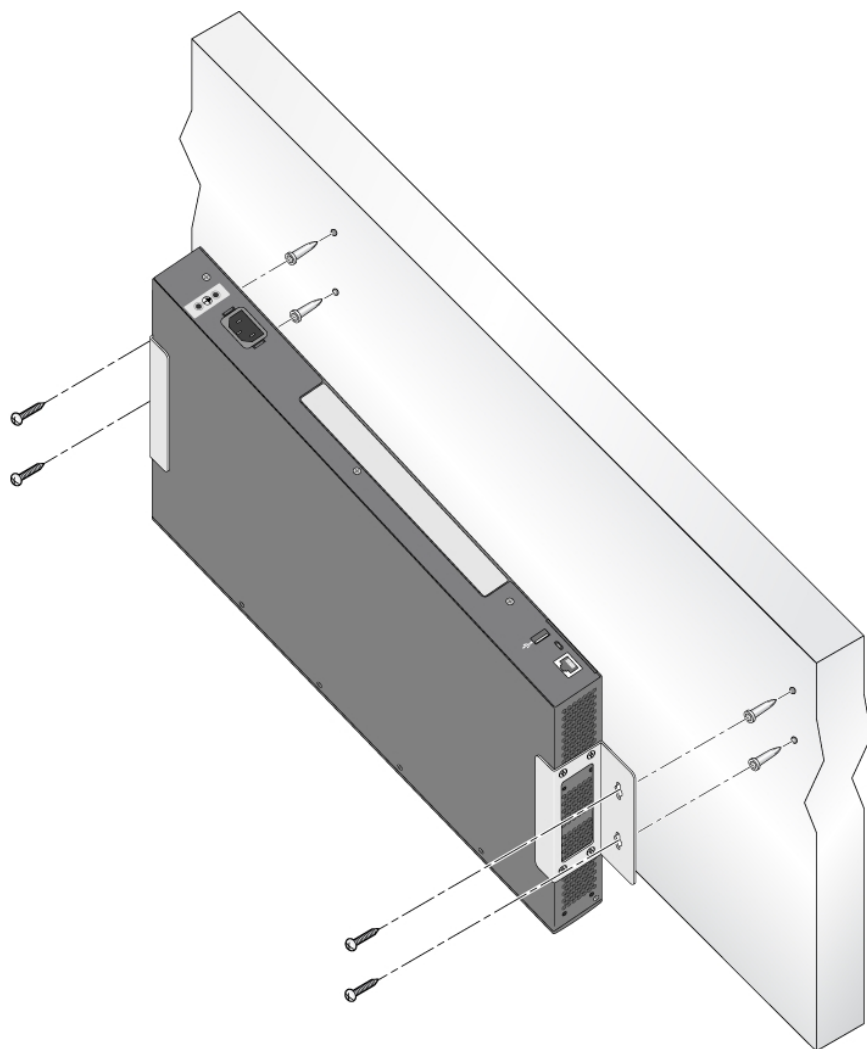
图 13: 壁式安装
